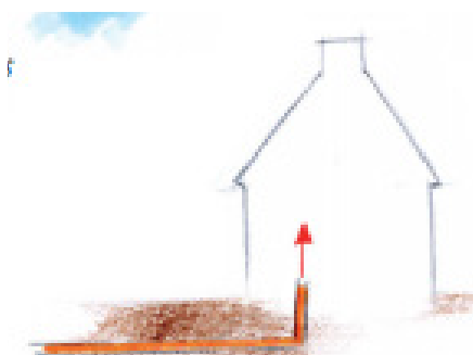
Principe du puits canadien pour préchauffer l'air entrant, ou le refroidir en été.
