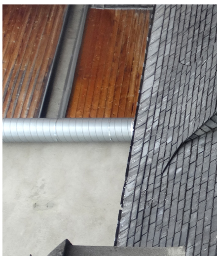
Toiture à croupe, couverture ardoise, houteau de ventilation, lucarne à croupe «capucine».
