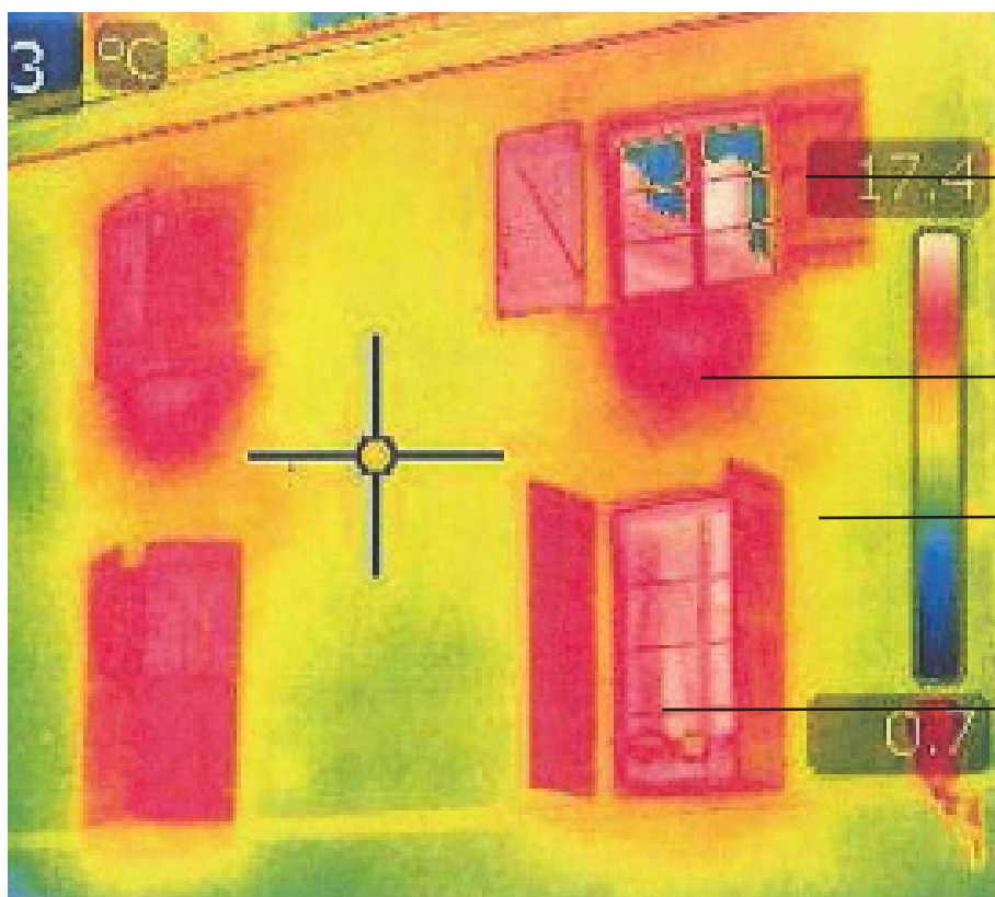
Déperditions thermiques des fenêtres mises en évidence par la thermographie. L'allège de la baie est un poste de déperdition important à ne pas négliger. Source : Oliva/Courgey, l'Isolation Thermique Ecologique. Source : L'isolation thermique écologique, Oliva/Courgey;
