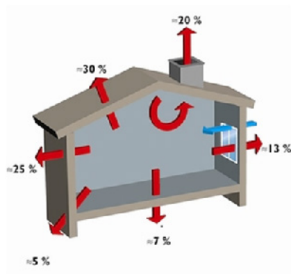
Schéma déperditions toiture
