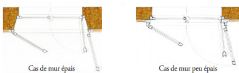
Quelques exemples d'application de joint à calfeutrement à queue d'aronde en silicone pour rétablir l'étanchéité des menuiseries.. Source : documentatgion technique Flexisol.
